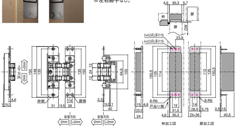
IDH-20 (隠し丁番本体) ※左右勝手なし。 枠側取付ベース
